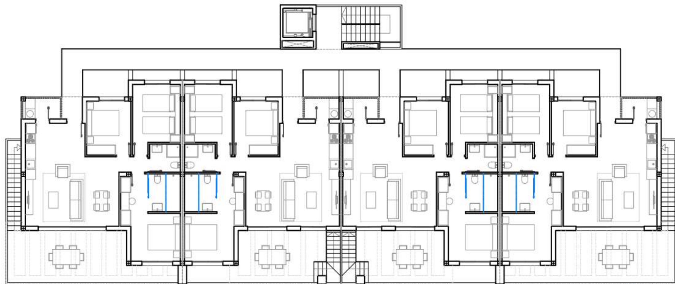
PLANTA ÁTICO
